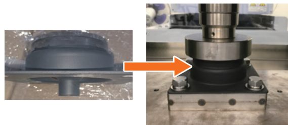
□ 防振ゴムの圧縮試験の様子
