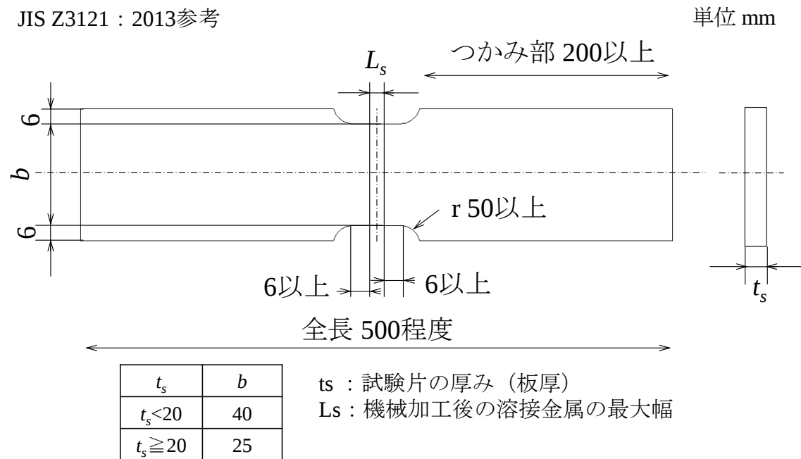
図 1 1 号試験片_引張試験片
