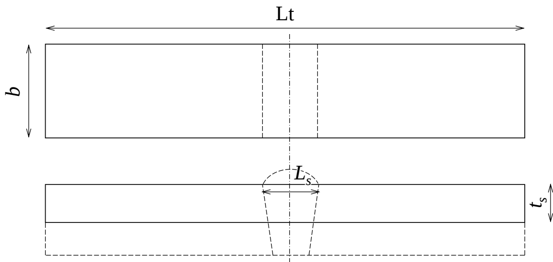
図2 表曲げ試験片
