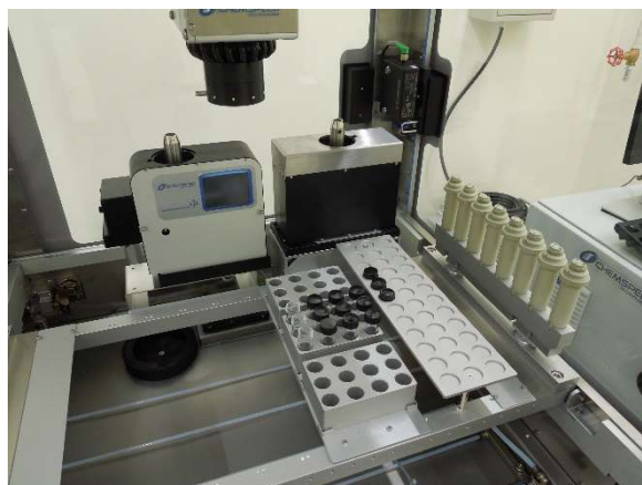
図 2. FLEX POWDERDOSE の内部
